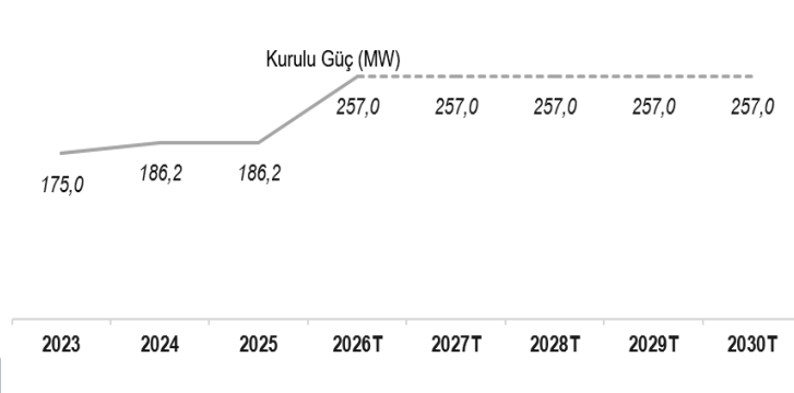
Grafik 3: Elmacık RES'in 2026 yılında devreye girmesi ile kurulu gücün 186,2 MW'den 257,0 MW'ye çıkması öngörülmekte
