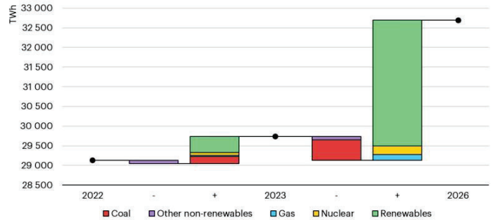
Küresel Elektrik Üretimindeki Değişimler, 2022-2026
