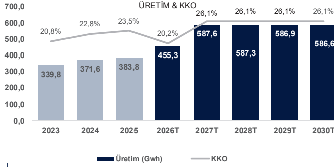
Grafik 4: 2025 yılında ortalama KKO %23,5 olarak gerçekleşirken, bu oranın 2026 yılında Elmacık RES'in kısmen devreye olması nedeniyle %20,2 seviyesine gerilemesi ve söz konusu santralin tam randımanlı faaliyete geçmesi ile 2027 yılında %26,1 seviyesine çıkması öngörülmekte
